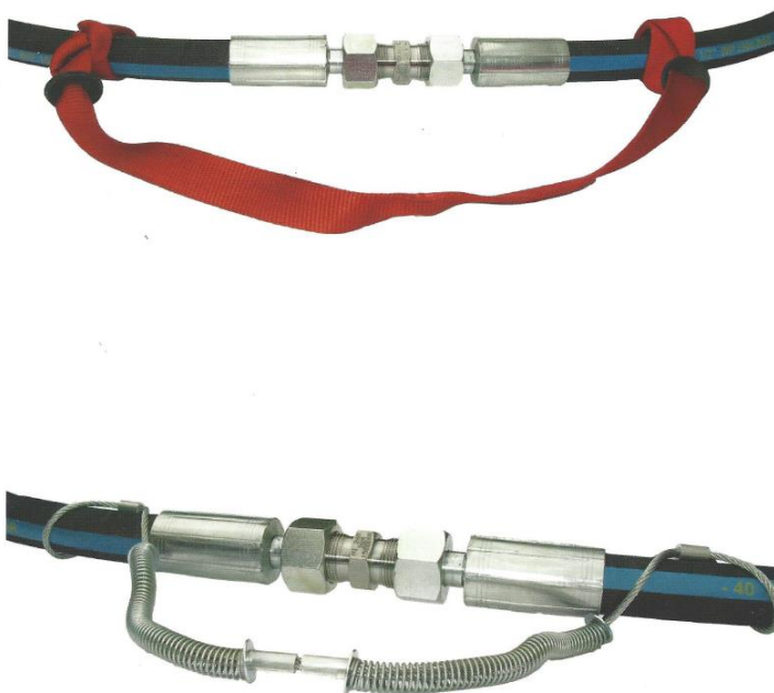
Figuur 3: voorbeeld van slangbreuk beveiligingen
